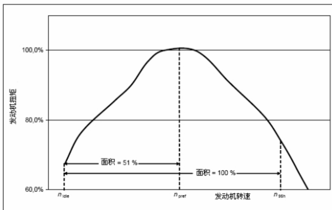
图 C.6 参考转速 ( n_{pref} ) 的确定
