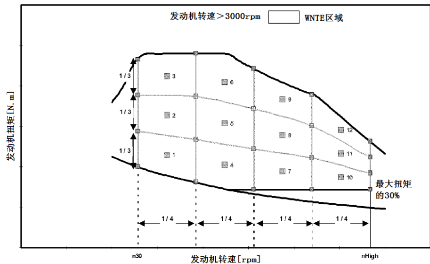
图 E.6 WNTe 试验网格 (发动机额定转速 > 3000rpm)
