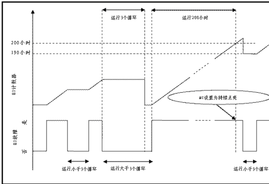
图 F.4 BI 计数器激活原理说明
