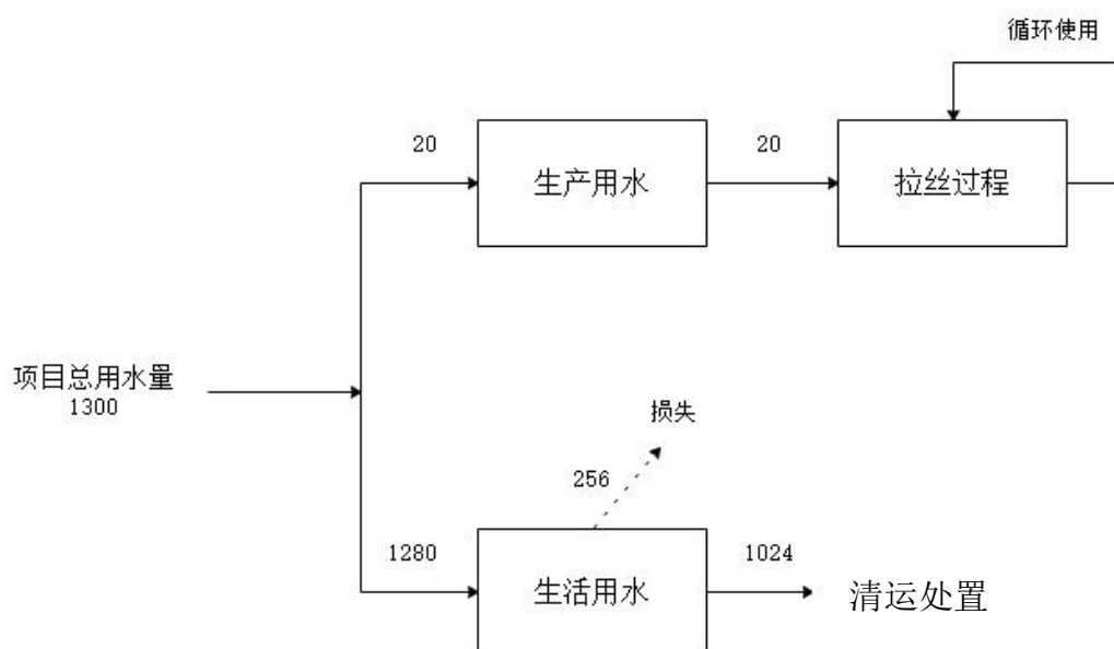
图 3-4 项目水平衡图 (单位: t/a)
