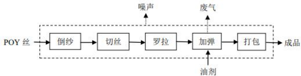
图 3-5 DTY 丝生产工艺流程图
