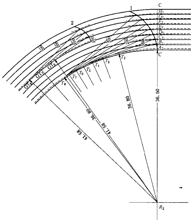
1——1 000 m、3 000 m 和 5 000 m 的起点线； 2——1 000 m、3 000 m 和 5 000 m 的分组起跑线。 注：R 2 C——36.50 m；R 2 A T ——36.80 m；R 2 B T ——36.80 m + 1.12 m；R 2 G T ……H T ——37.92 m + 每道 1.22 m； T 2 T 8 ——切线点；G 1 G 8 ——分组起跑线的切线点。
