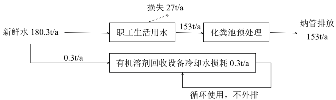
图 3-4 本项目水平衡图
