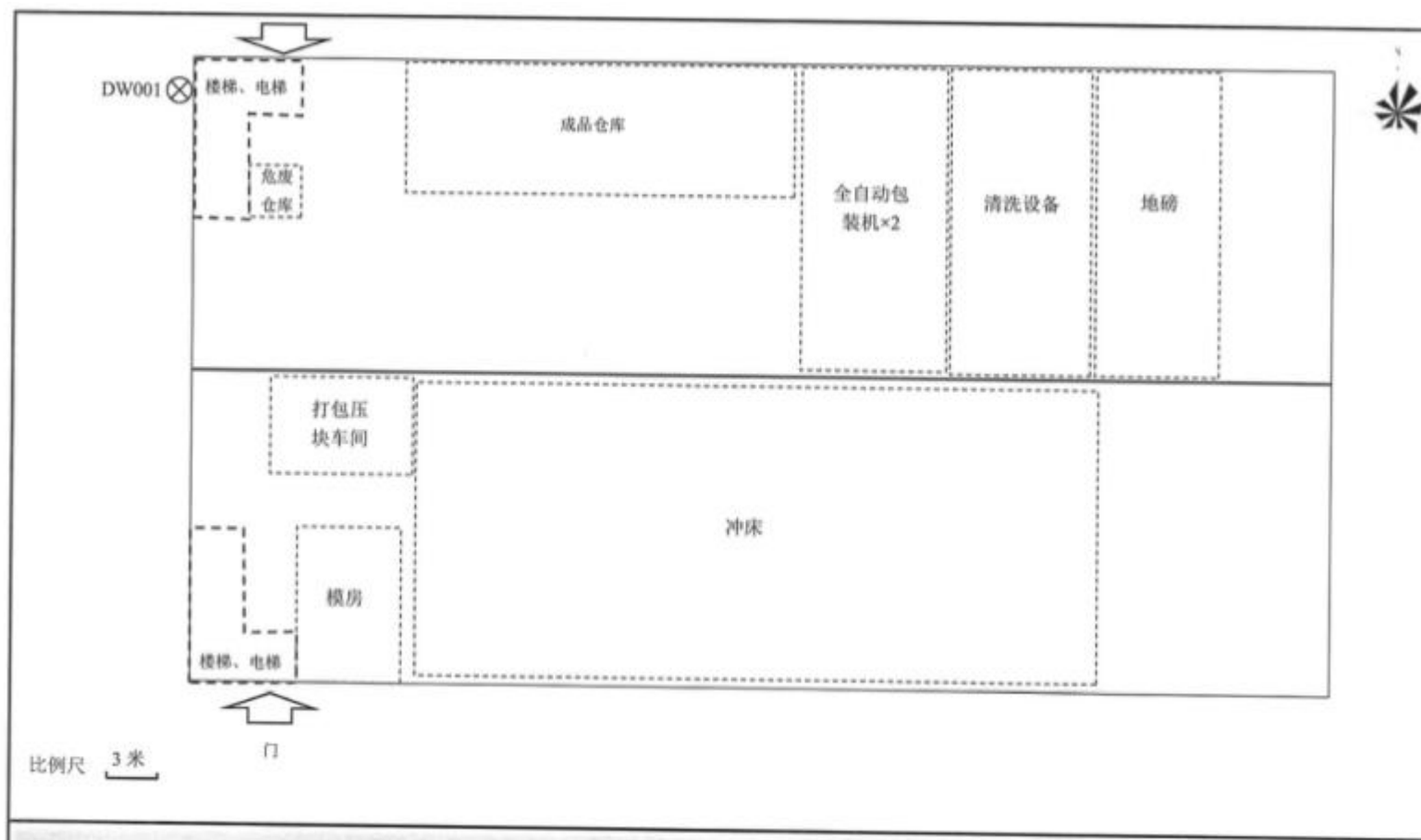
图 3-3 本项目厂区平面布置图
