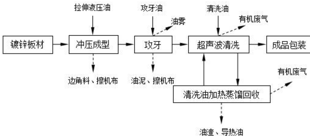
图 3-5 本项目各系列机壳生产工艺流程及产污环节示意图
