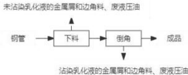
图 3-5 本项目链条套筒、链条滚子生产工艺流程及产污环节示意图
