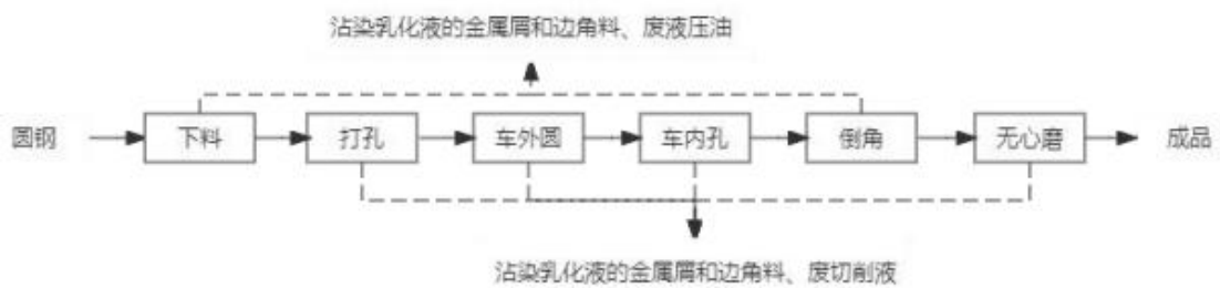
图 3-6 本项目链条插轴生产工艺流程及产污环节示意图
