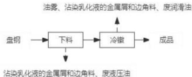
图 3-7 本项目链条插轴生产工艺流程及产污环节示意图
