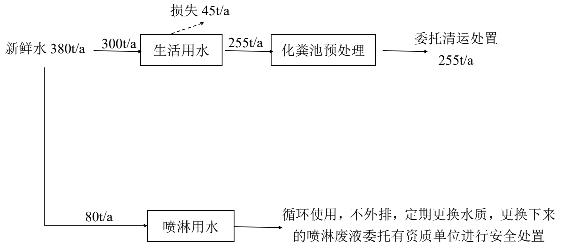
图 3-4 本项目水平衡图
