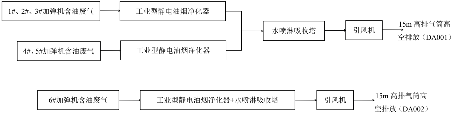
图 4-2 本项目废气处理工艺流程
