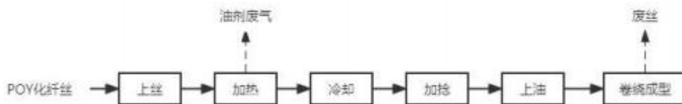
图 3-4 化纤丝加弹生产工艺及产污流程图
