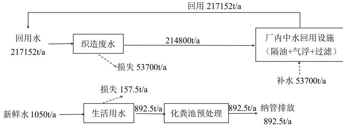
图 3-3 本项目水平衡图
