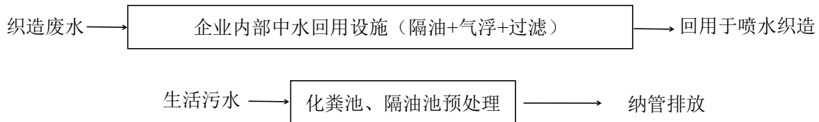
图 4-1 项目生活污水处理工艺流程图
