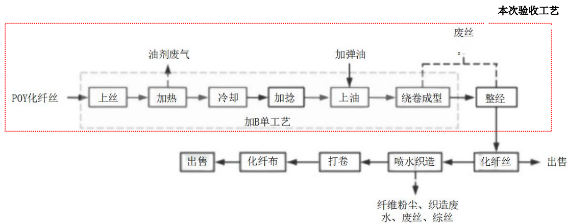
图 3-4 本项目各类纺织面料生产工艺及产污流程图
