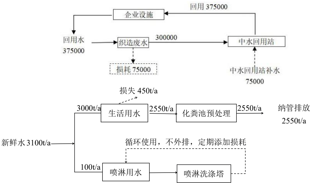
图 3-3 本项目水平衡图
