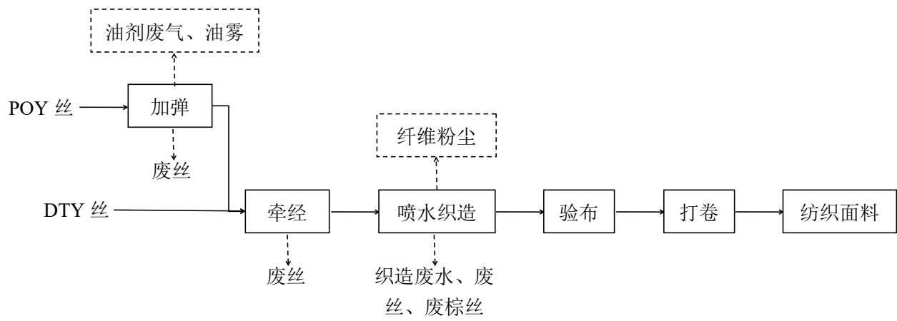
图 3-4 本项目高端纺织面料生产工艺及产污流程图
