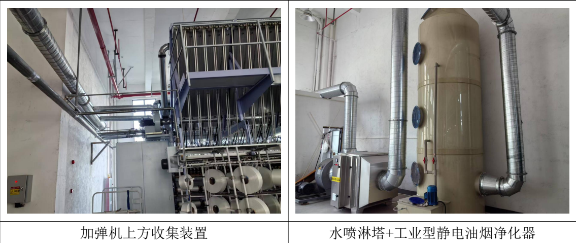
图 4-3 本项目废气、废水处理设施照片
