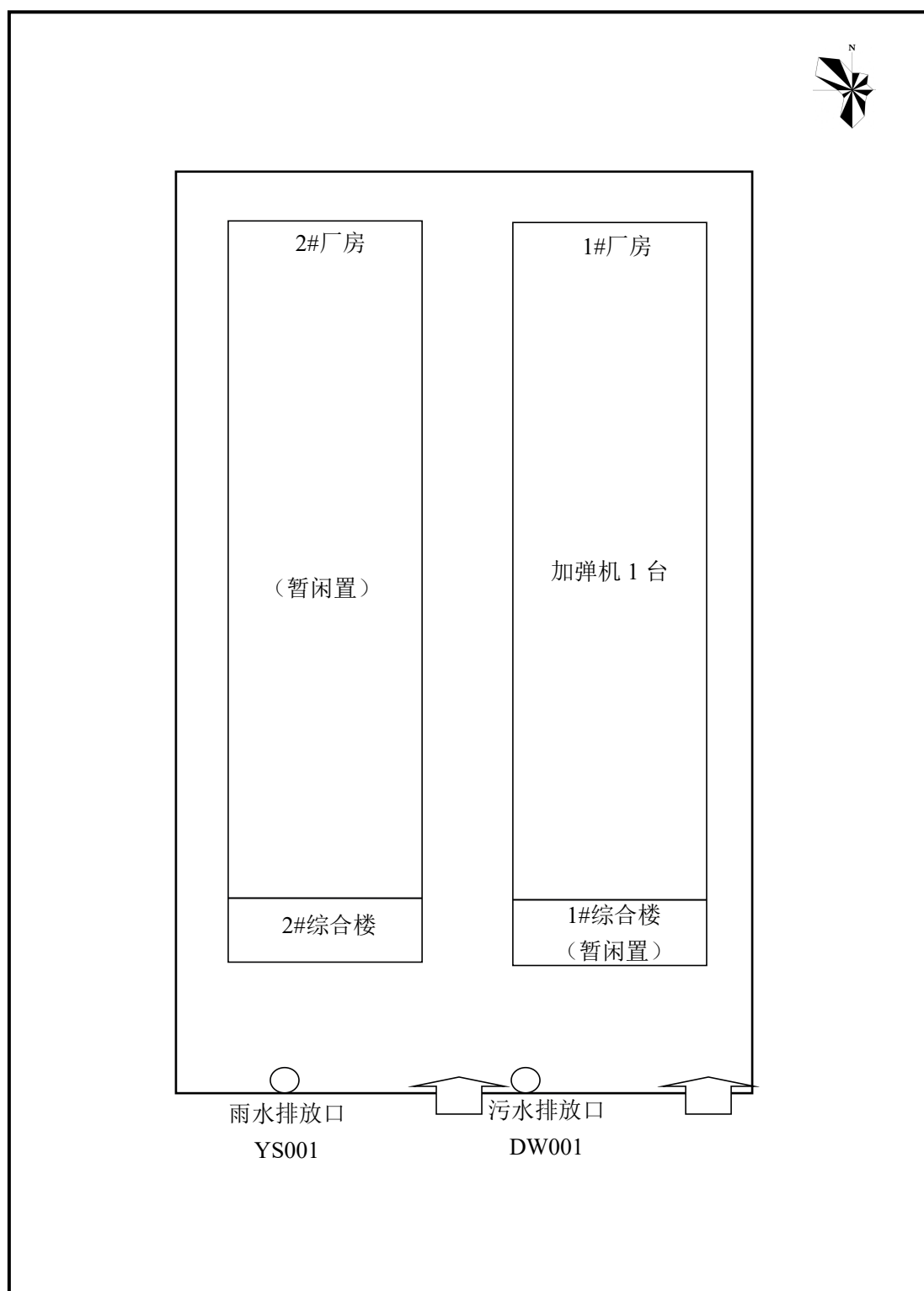
图 3-2 本项目厂区平面布置图（2 楼）
