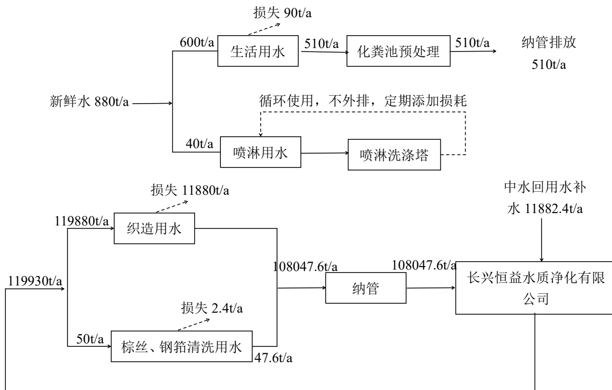
图 3-3 本项目水平衡图
