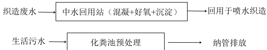
图 4-1 项目生活污水处理工艺流程图
