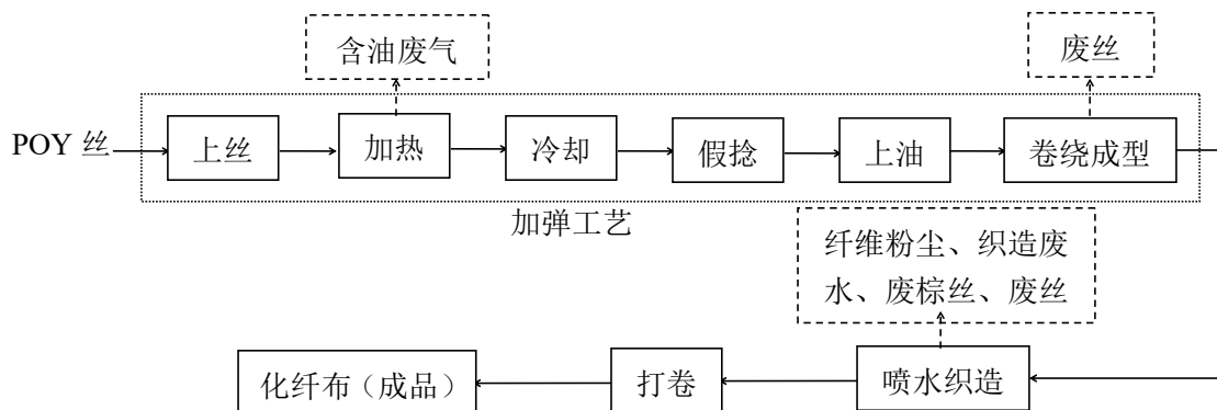
图 3-4 本项目化纤丝生产工艺及产污流程图
