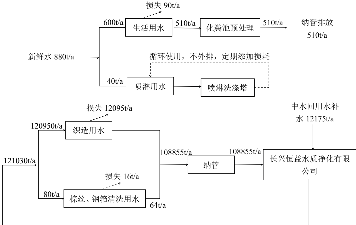
图 3-4 本项目水平衡图
