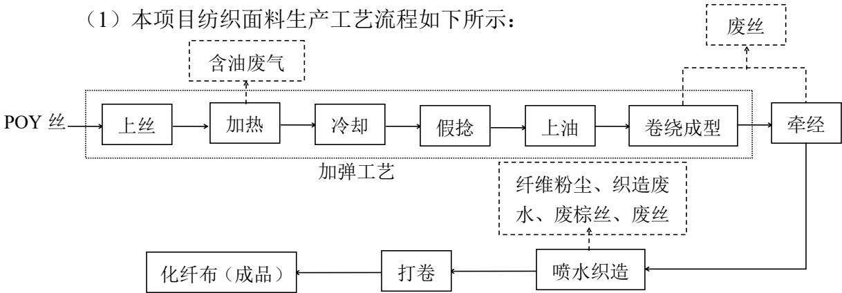
图 3-5 本项目化纤丝生产工艺及产污流程图
