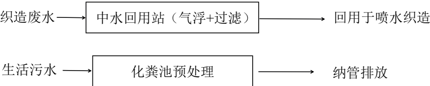
图 4-1 项目生活污水处理工艺流程图
