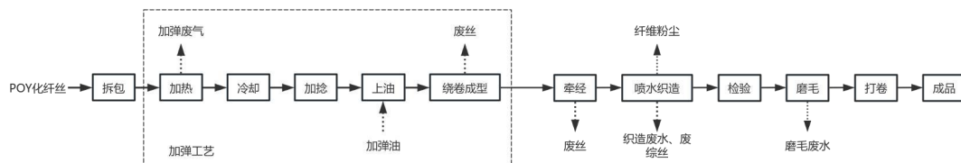
图 3-4 本项目高档功能性纺织面料生产工艺及产污流程图
