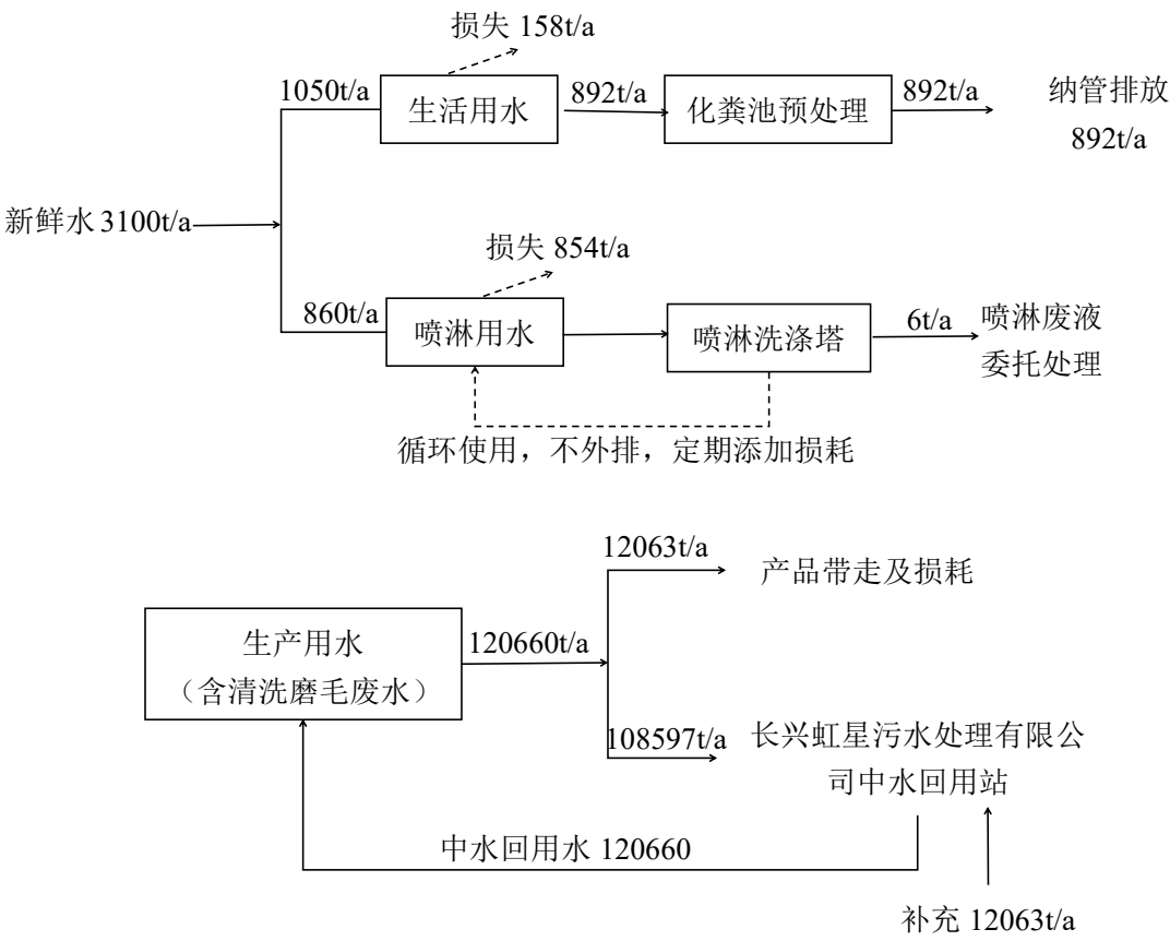
图 3-3 本项目水平衡图
